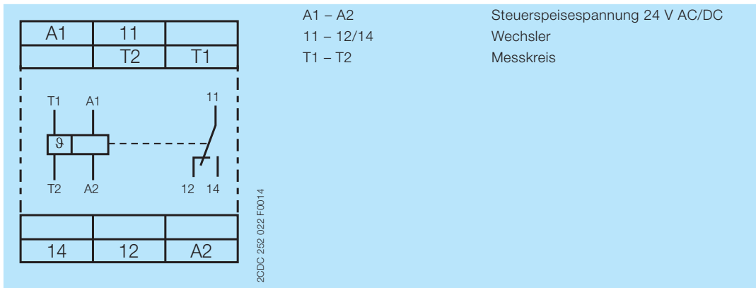
Anschlussbild CM-MSS.12
