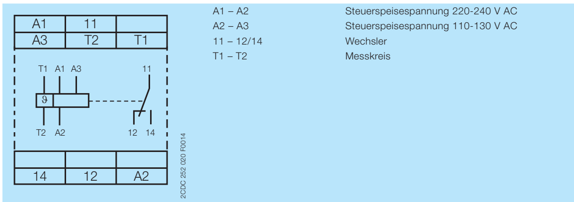
Anschlussbild CM-MSS.13
