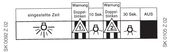
Warnfunktion beim E 232 E-8/230 Plus
