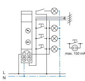
E232 E-230 Multi 10 4-Leiter
