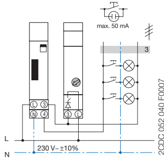
E232 HLM 3-Leiter
