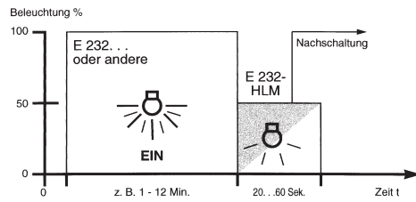
Zeitablauf Treppenlicht-Zeitschalter mit Halblichtmodul E 232 HLM
