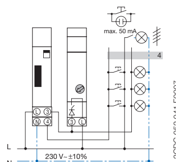
E232 HLM 4-Leiter
