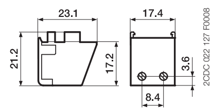
integrierter Hilfskontakt
