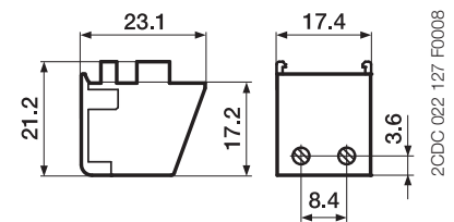
integrierter Hilfskontakt
