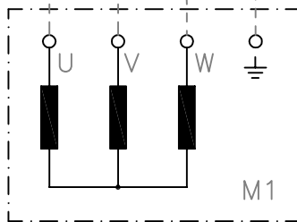
Sternverschaltung
