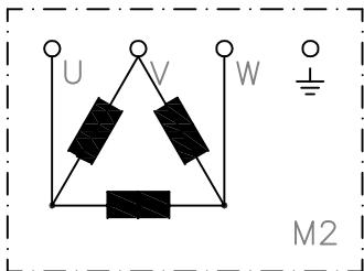
Dreieckverschaltung
