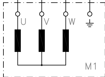
Sternverschaltung
