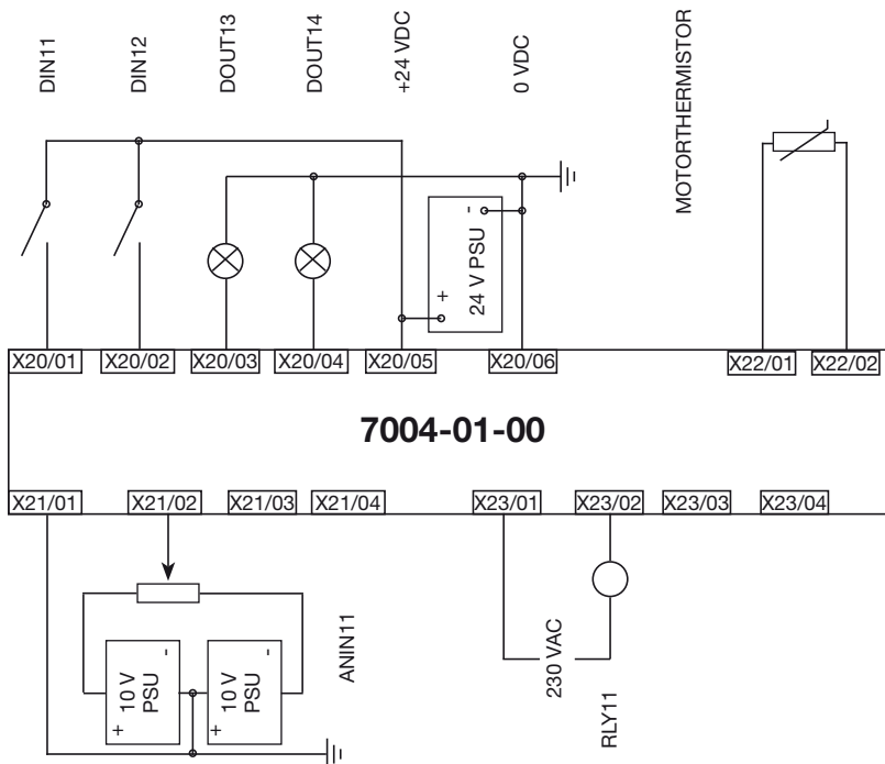
Beispielverdrahtung für GPIO Modul 7004-01-00
